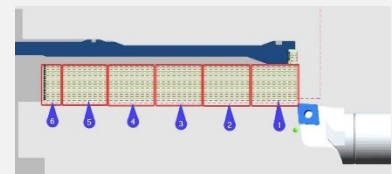
Lastunkatkoja vakiosyvyydellä
