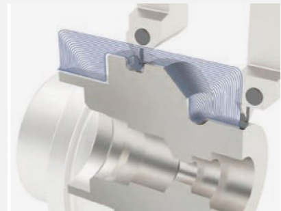
Adaptiivinen rouhintasorvaus
